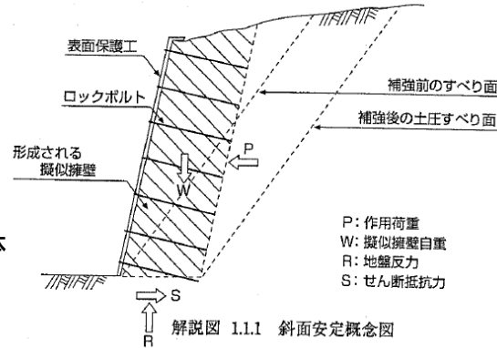
解説図 1.1.1 斜面安定概念図 出典:SW工法・TOP工法設計マニュアル
